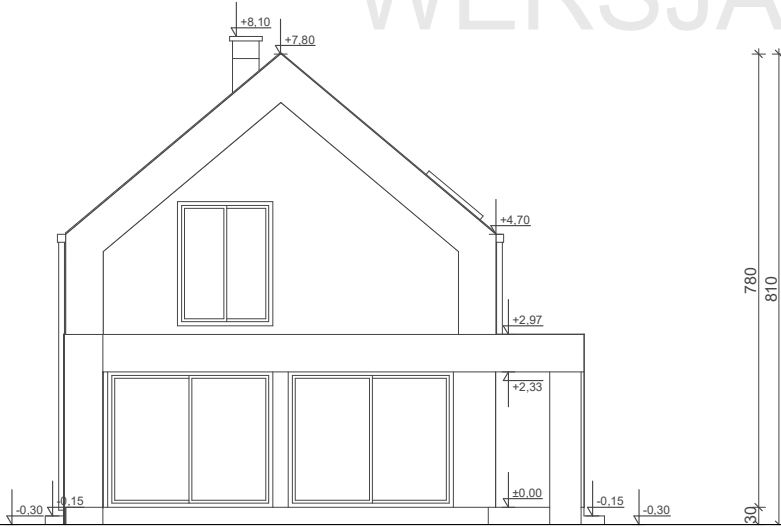
ELEWACJA FRONTOWA
