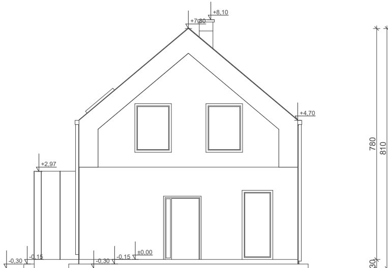
ELEWACJA OGRODOWA
