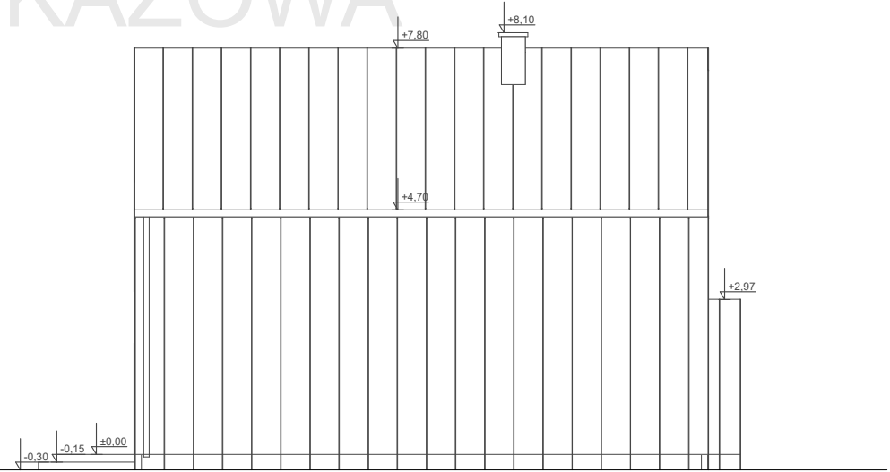
ELEWACJA BOK 1
