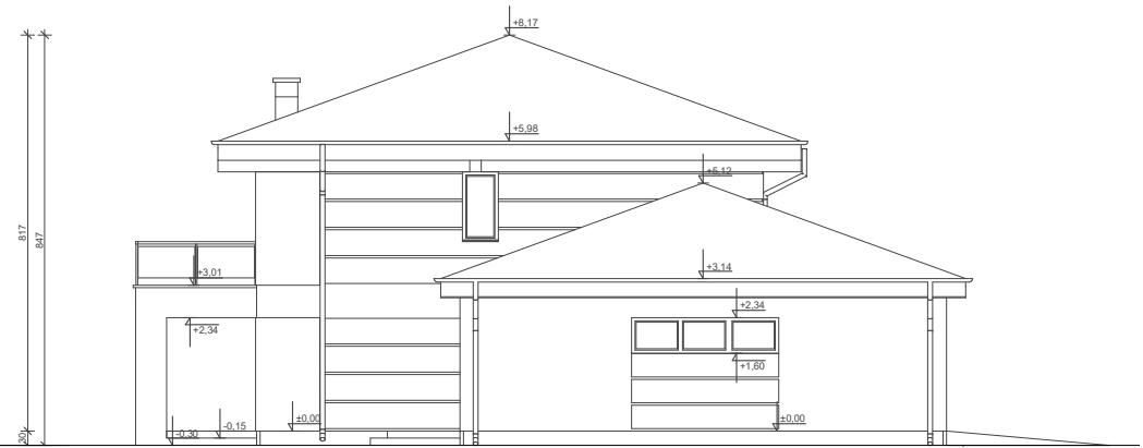
ELEWACJA BOK 1
