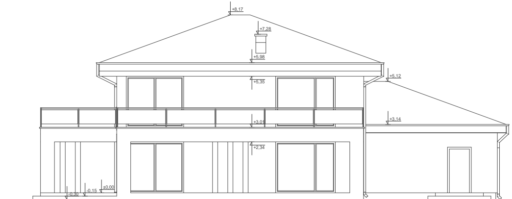
ELEWACJA OGRODOWA
