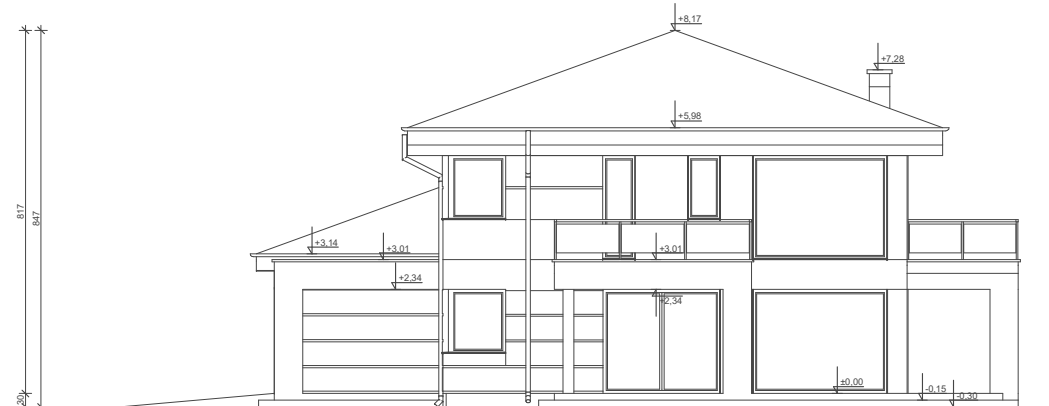
ELEWACJA BOK 2
