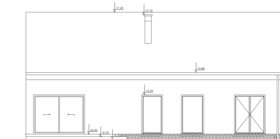
ELEWACJA OGRODOWA
