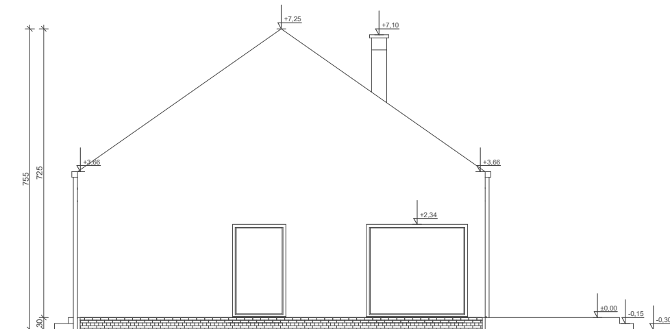
ELEWACJA BOK 2
