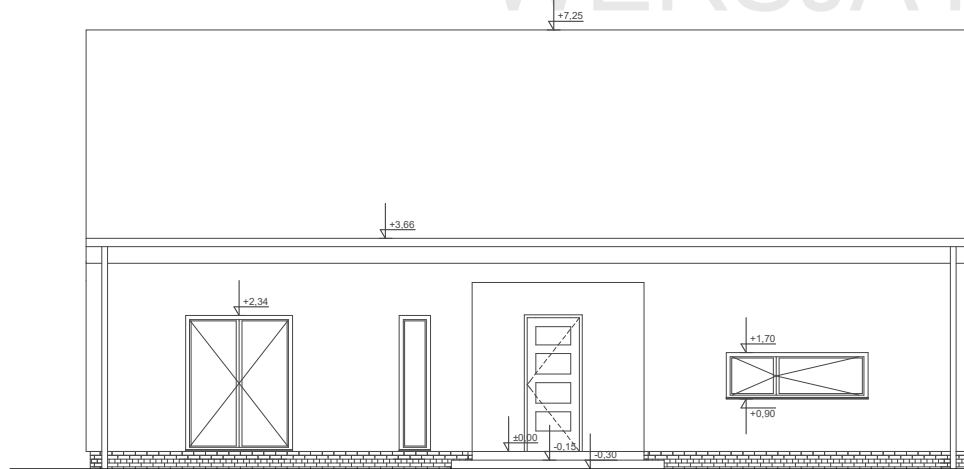
ELEWACJA FRONTOWA
