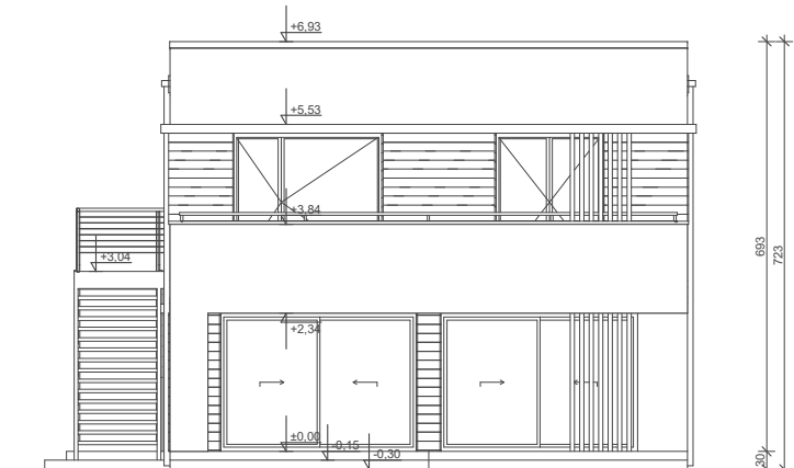
ELEWACJA OGRODOWA
