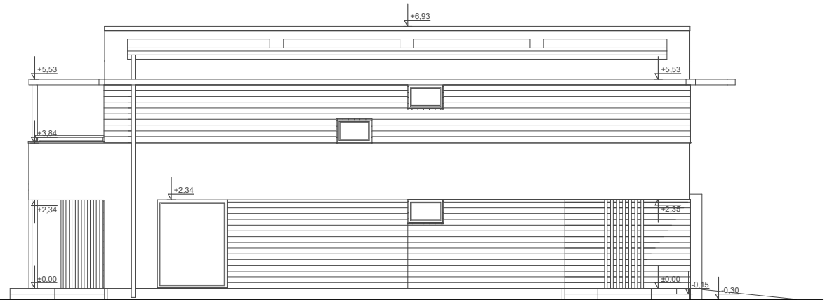
ELEWACJA BOK 1
