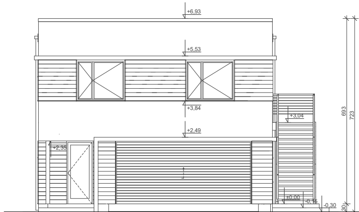
ELEWACJA FRONTOWA
