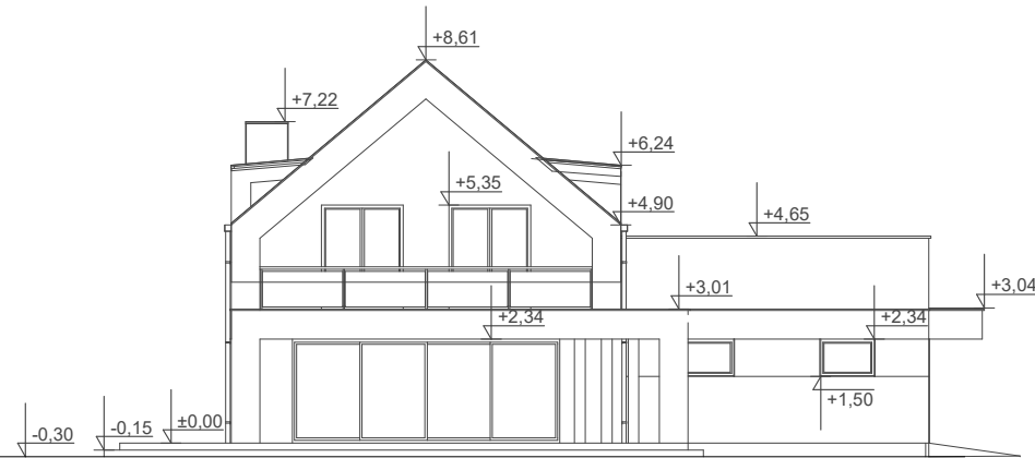
ELEWACJA BOK 1
