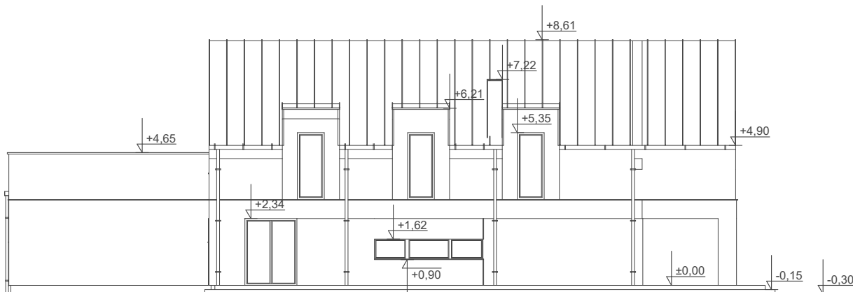
ELEWACJA OGRODOWA
