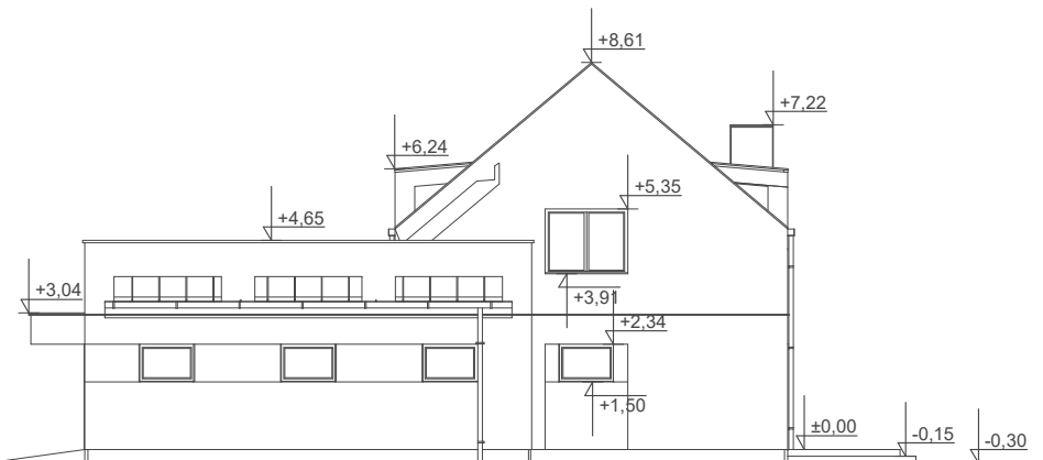
ELEWACJA BOK 2
