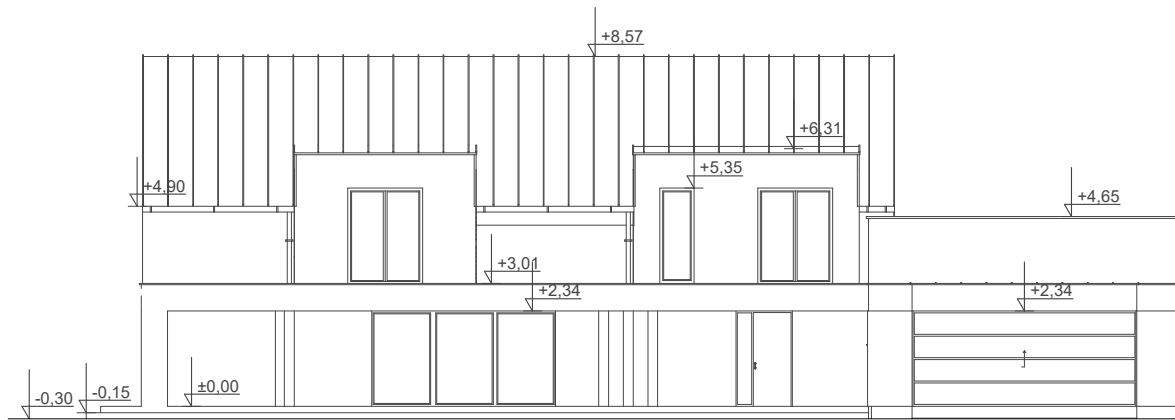
ELEWACJA FRONTOWA
