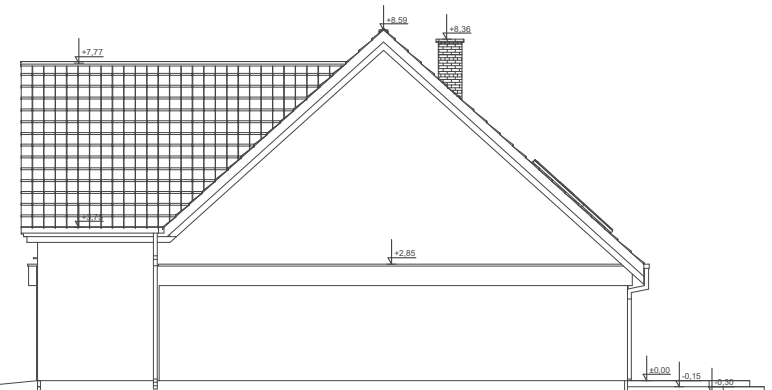
ELEWACJA BOK 2
