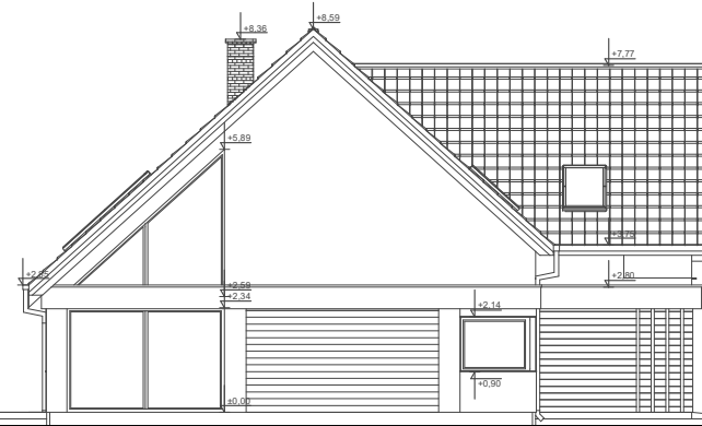
ELEWACJA BOK 1
