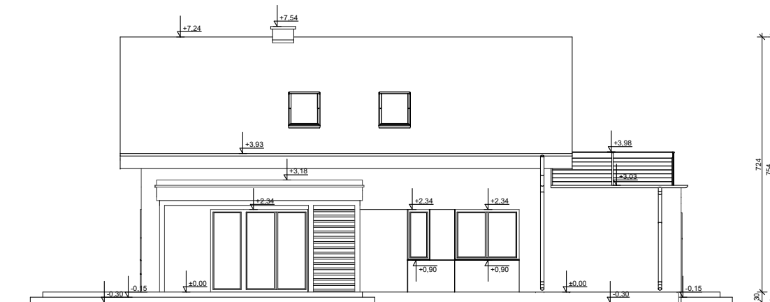
ELEWACJA OGRODOWA
