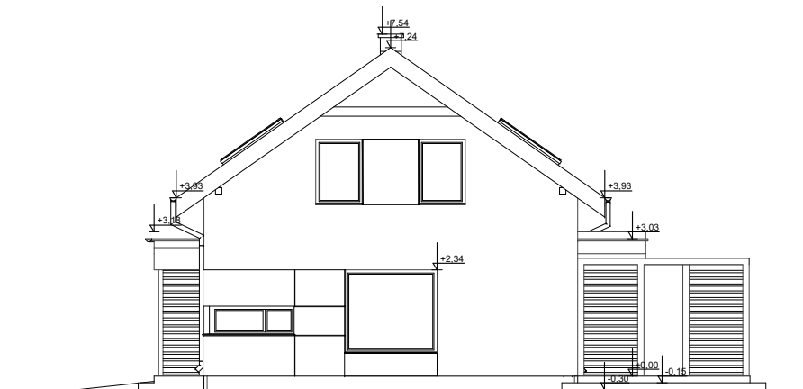
ELEWACJA BOK 2
