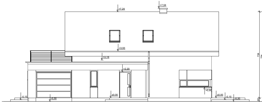
ELEWACJA FRONTOWA
