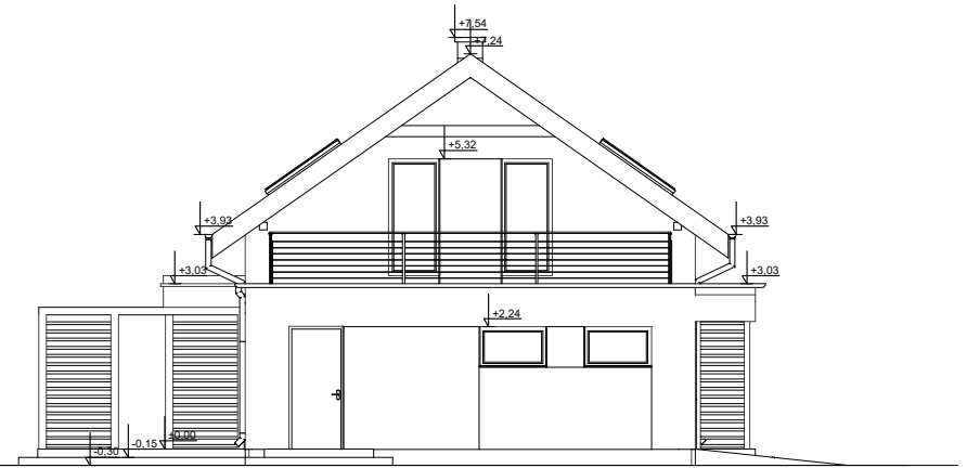
ELEWACJA BOK 1
