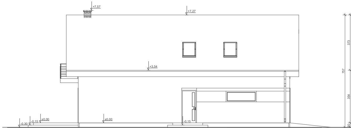
ELEWACJA FRONTOWA
