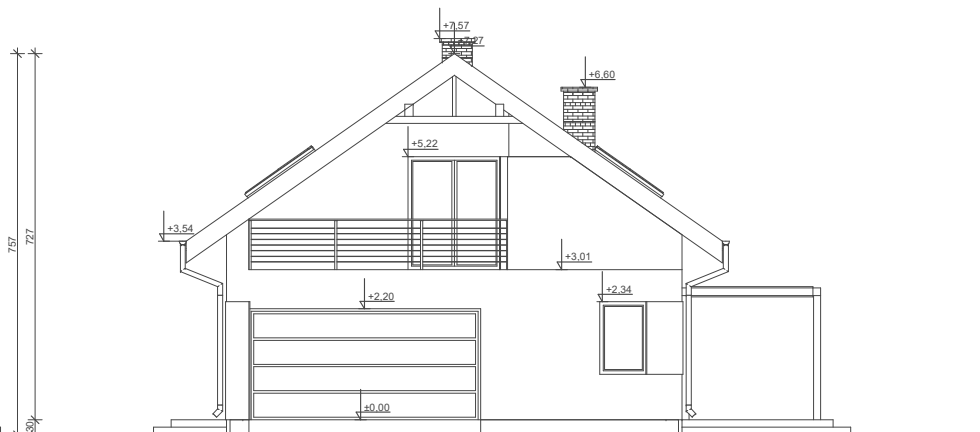
ELEWACJA BOK 2
