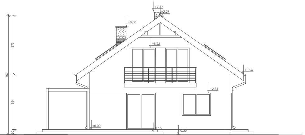
ELEWACJA BOK 1
