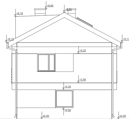
ELEWACJA BOK 2
