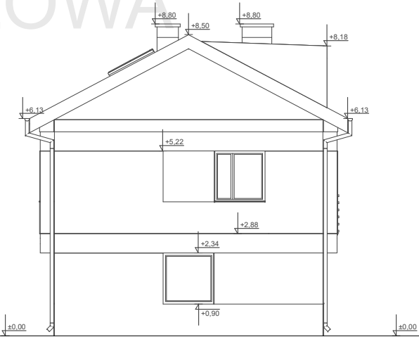
ELEWACJA BOK 1
