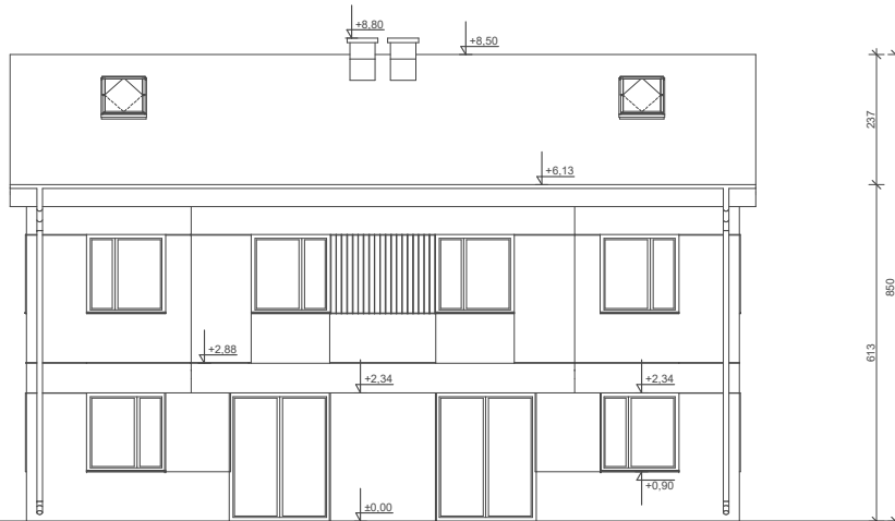
ELEWACJA OGRODOWA
