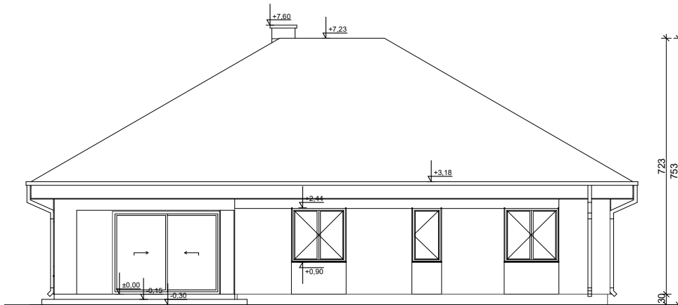
ELEWACJA OGRODOWA
