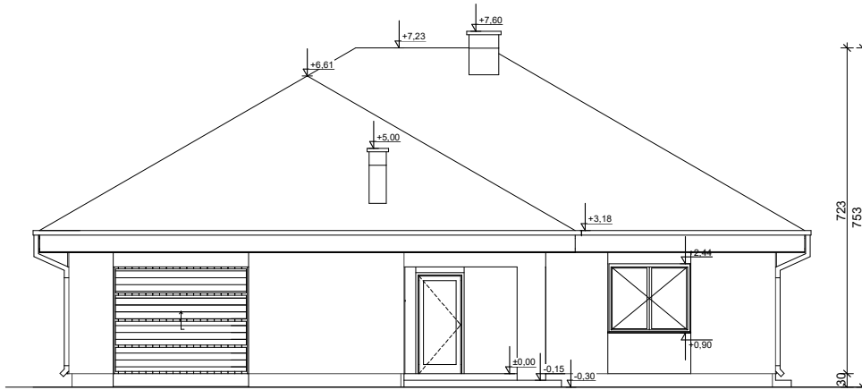
ELEWACJA FRONTOWA
