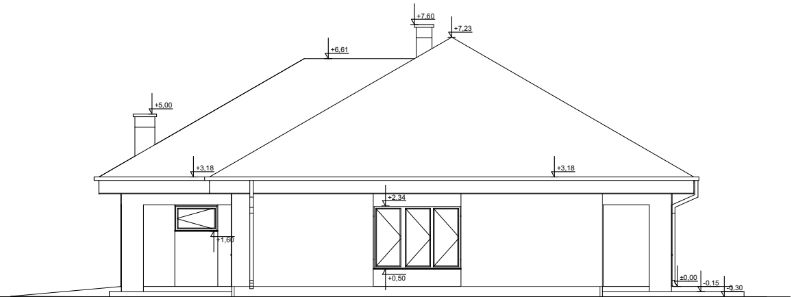
ELEWACJA BOK 2
