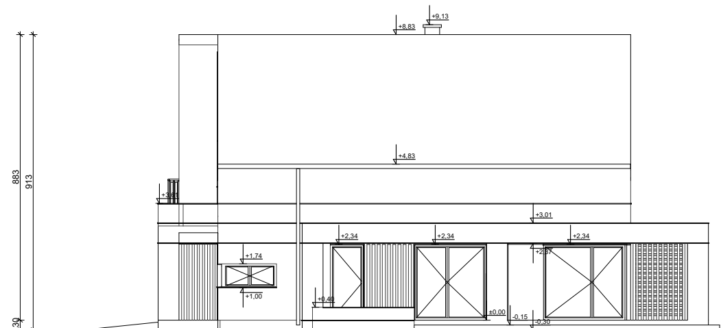
ELEWACJA BOK 2
