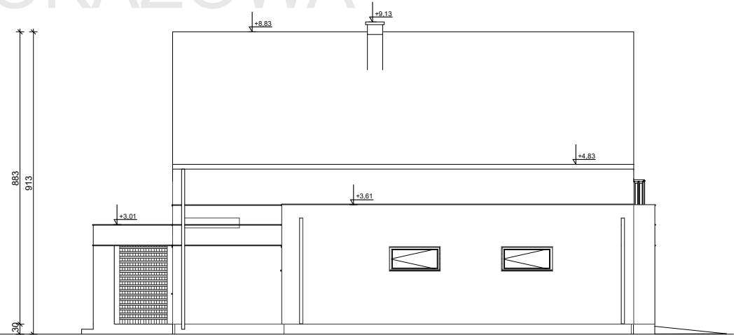
ELEWACJA BOK 1
