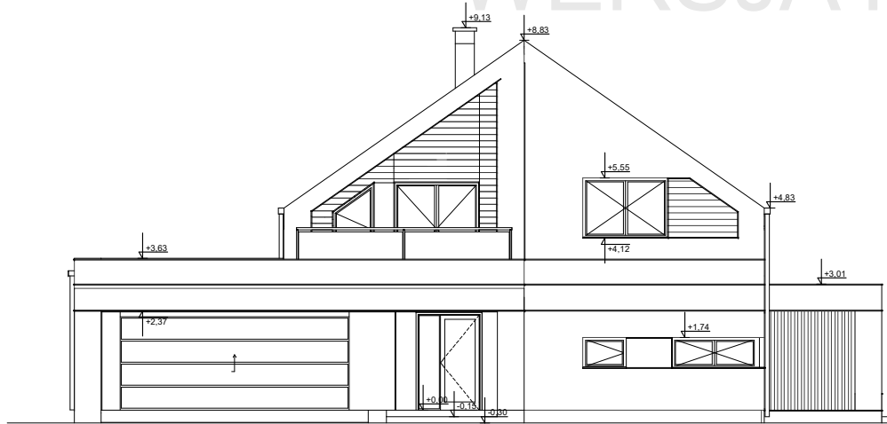
ELEWACJA FRONTOWA
