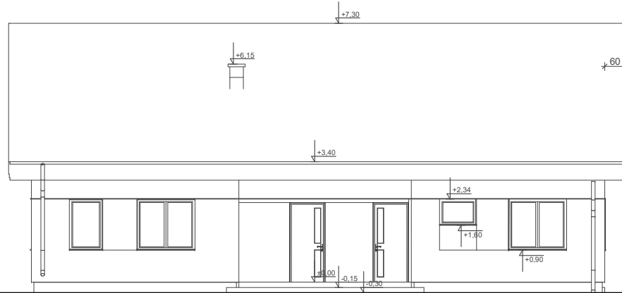
ELEWACJA FRONTOWA
