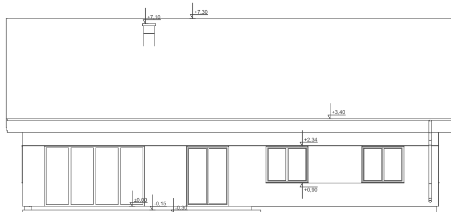
ELEWACJA OGRODOWA
