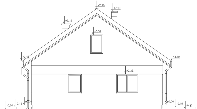
ELEWACJA BOK 1
