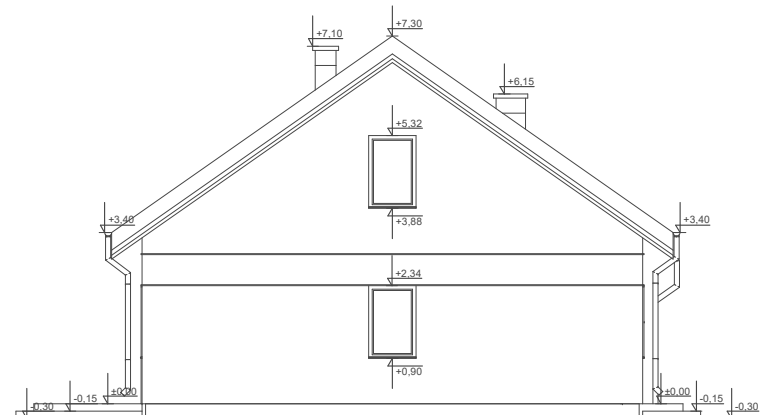
ELEWACJA BOK 2
