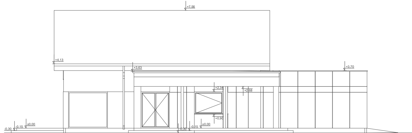
ELEWACJA BOK 1
