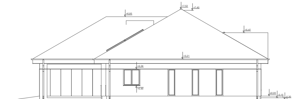
ELEWACJA BOK 2
