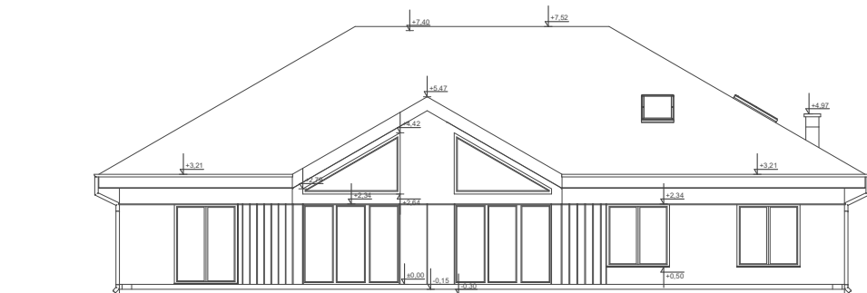
ELEWACJA OGRODOWA
