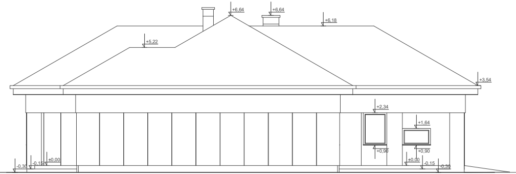
ELEWACJA BOK 1
