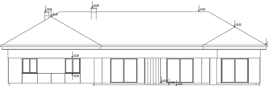
ELEWACJA OGRODOWA
