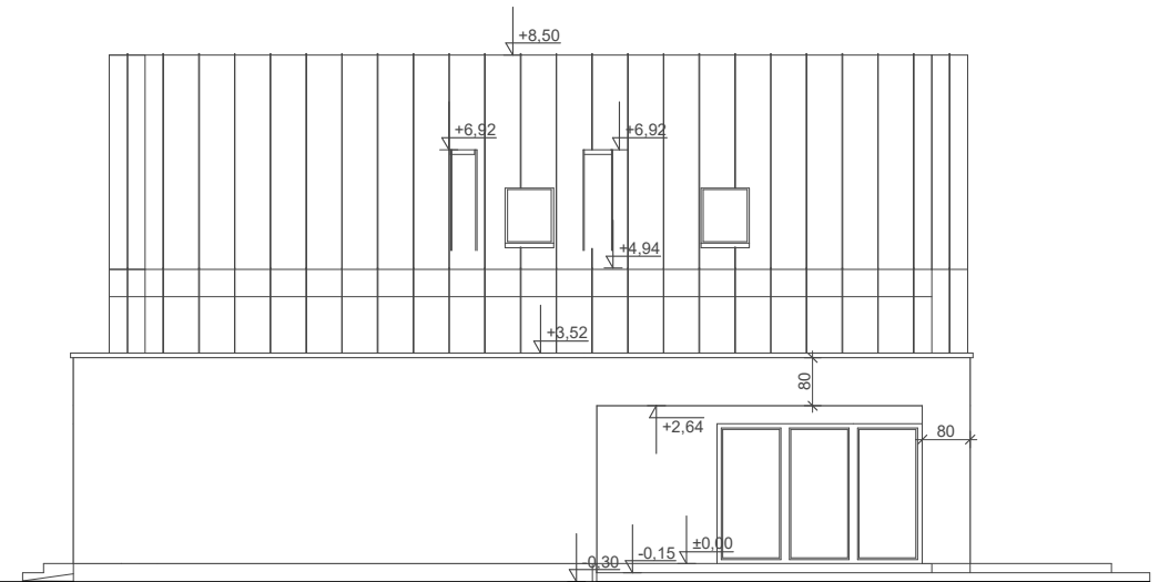
ELEWACJA BOK 2
