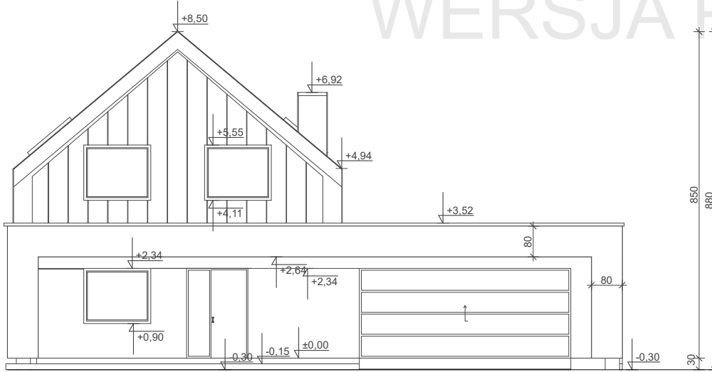
ELEWACJA FRONTOWA
