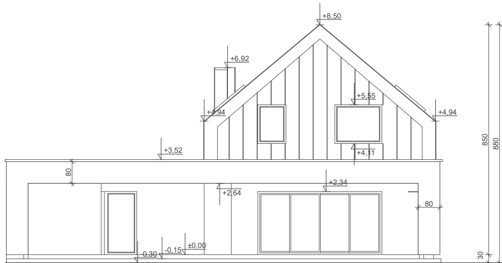
ELEWACJA OGRODOWA
