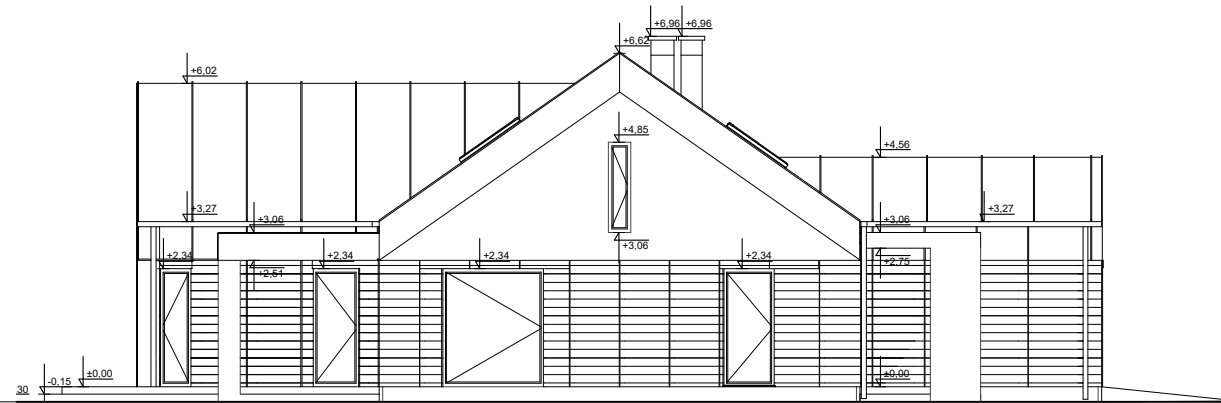
ELEWACJA BOK 1
