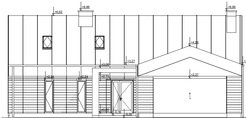
ELEWACJA FRONTOWA
