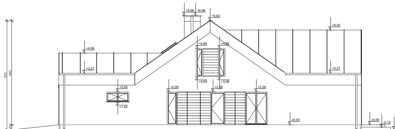
ELEWACJA BOK 2
