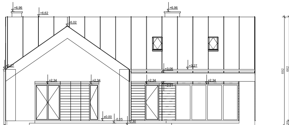
ELEWACJA OGRODOWA
