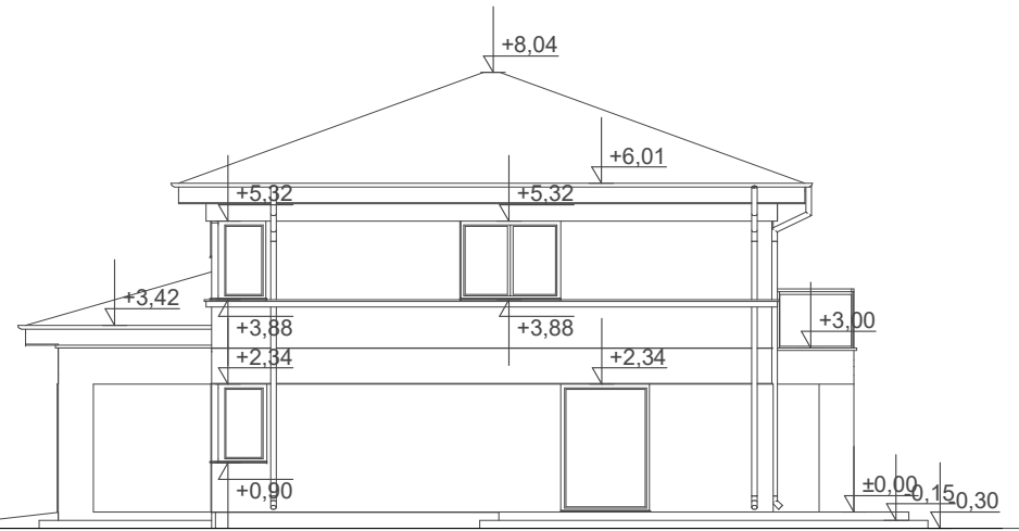
ELEWACJA BOK 1
