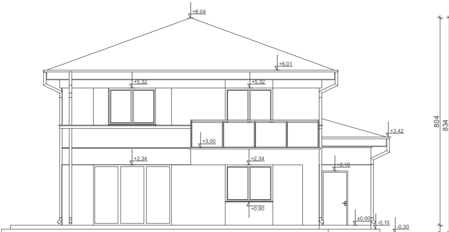
ELEWACJA OGRODOWA
