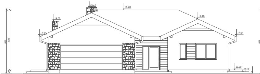
ELEWACJA FRONTOWA
