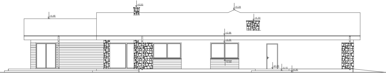
ELEWACJA BOK 1
