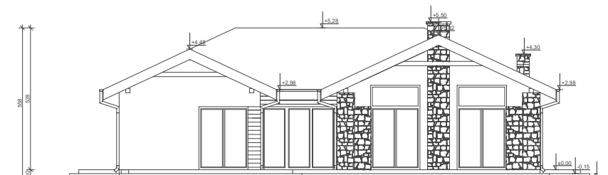
ELEWACJA OGRODOWA
