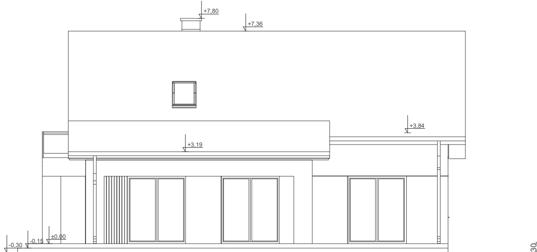
ELEWACJA OGRODOWA
