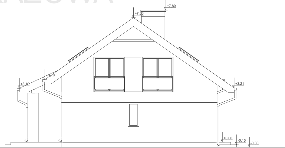
ELEWACJA BOK 1
