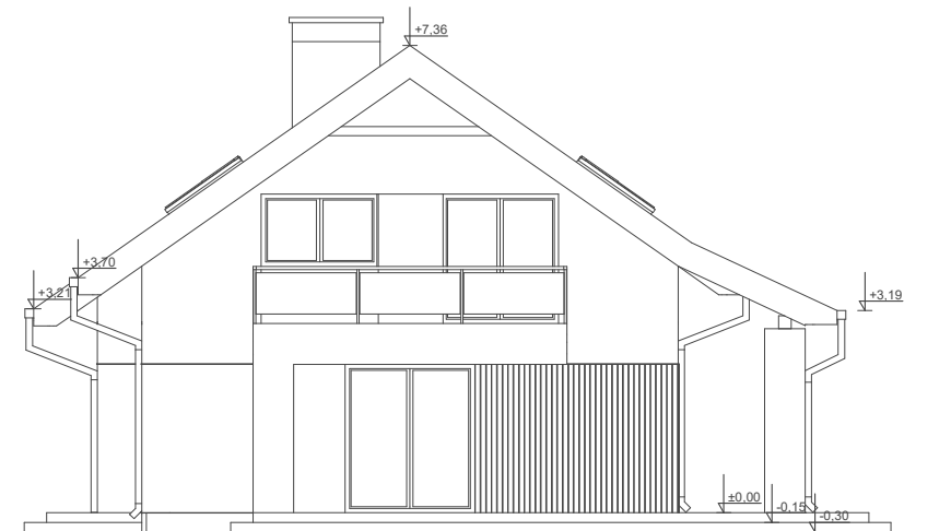
ELEWACJA BOK 2
