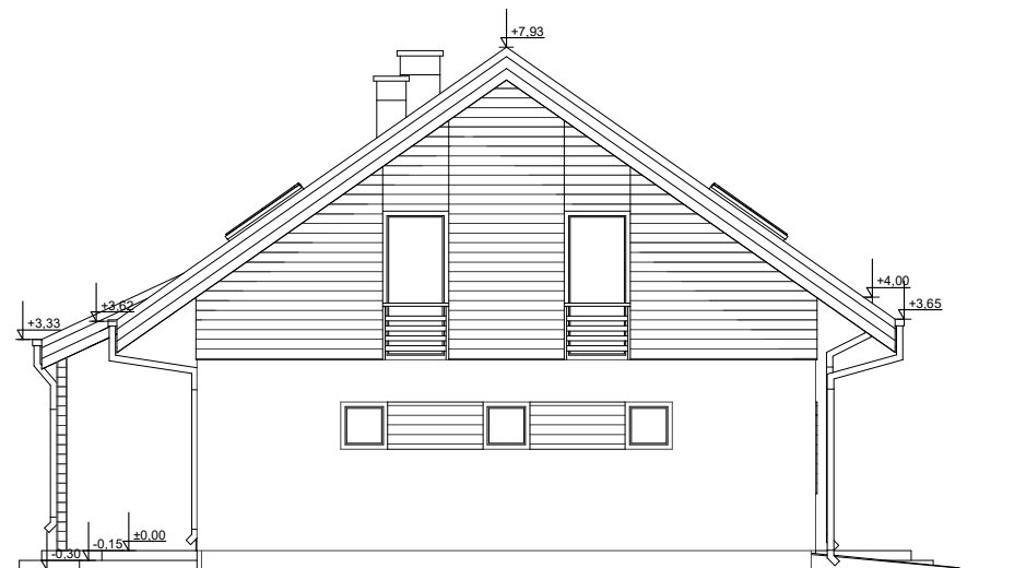
ELEWACJA BOK 2
