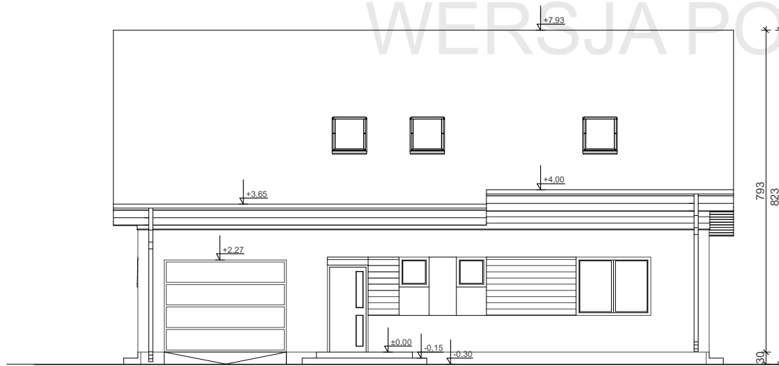
ELEWACJA FRONTOWA
