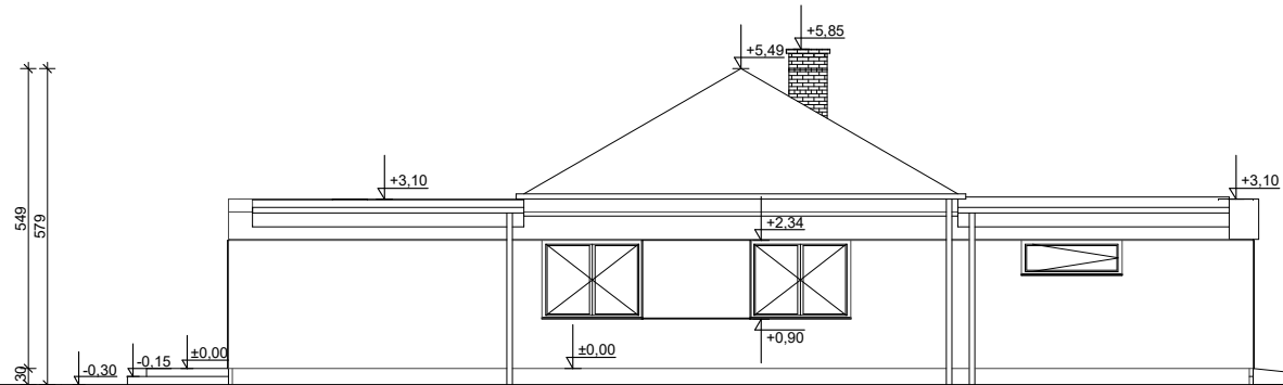
ELEWACJA BOK 1
