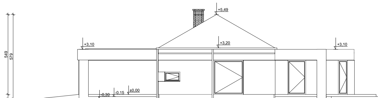
ELEWACJA BOK 2
