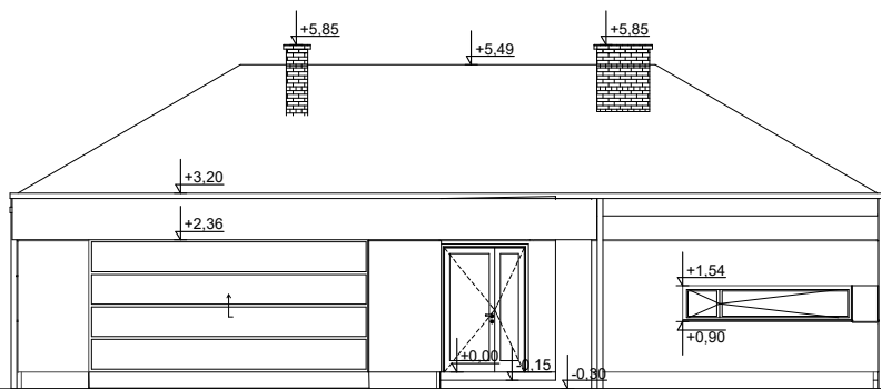
ELEWACJA FRONTOWA
