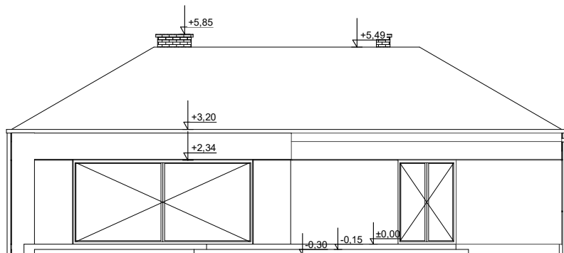
ELEWACJA OGRODOWA
