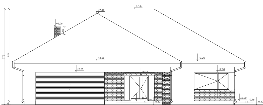
ELEWACJA FRONTOWA
