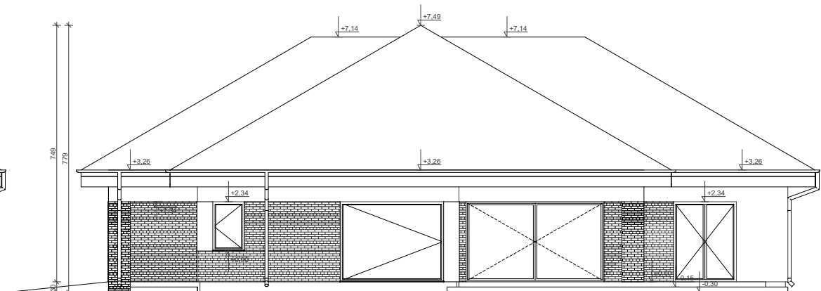
ELEWACJA BOK 2
