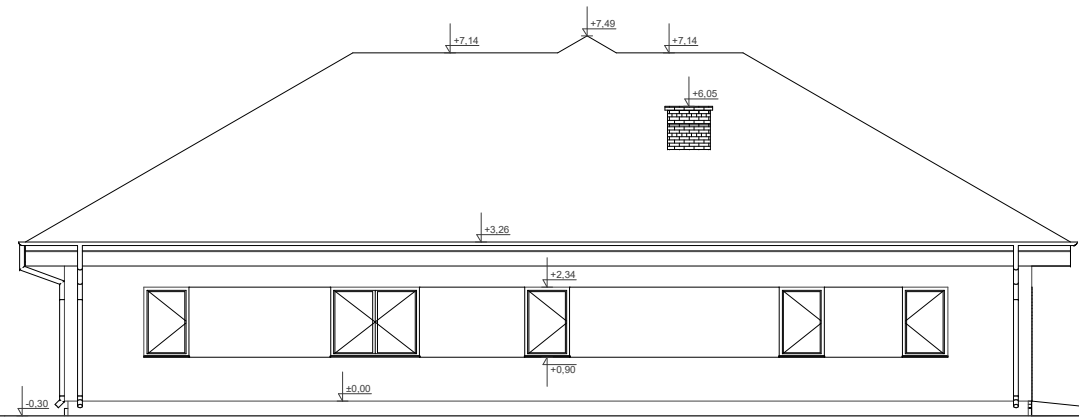
ELEWACJA BOK 1
