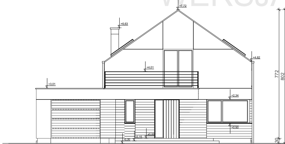
ELEWACJA FRONTOWA
