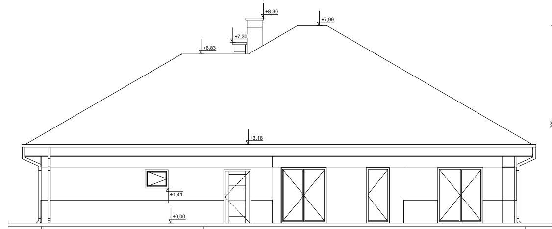
ELEWACJA BOK 2
