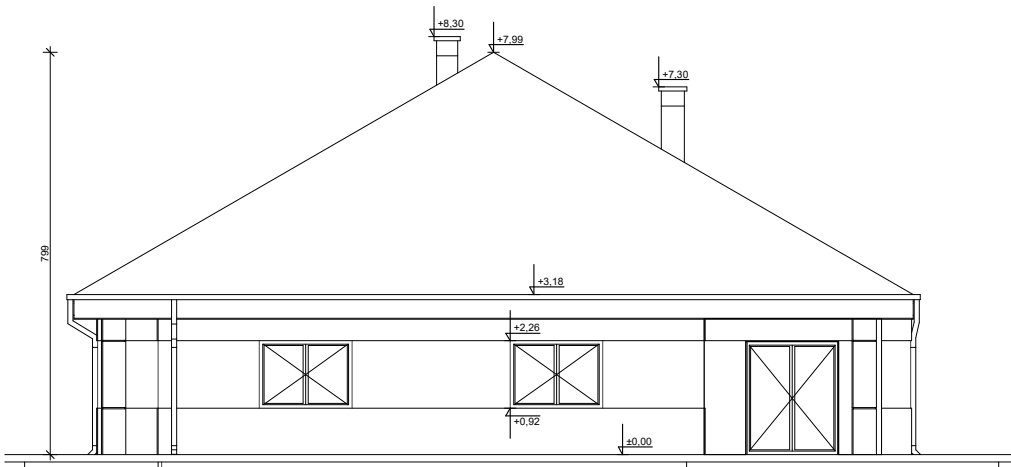
ELEWACJA OGRODOWA
