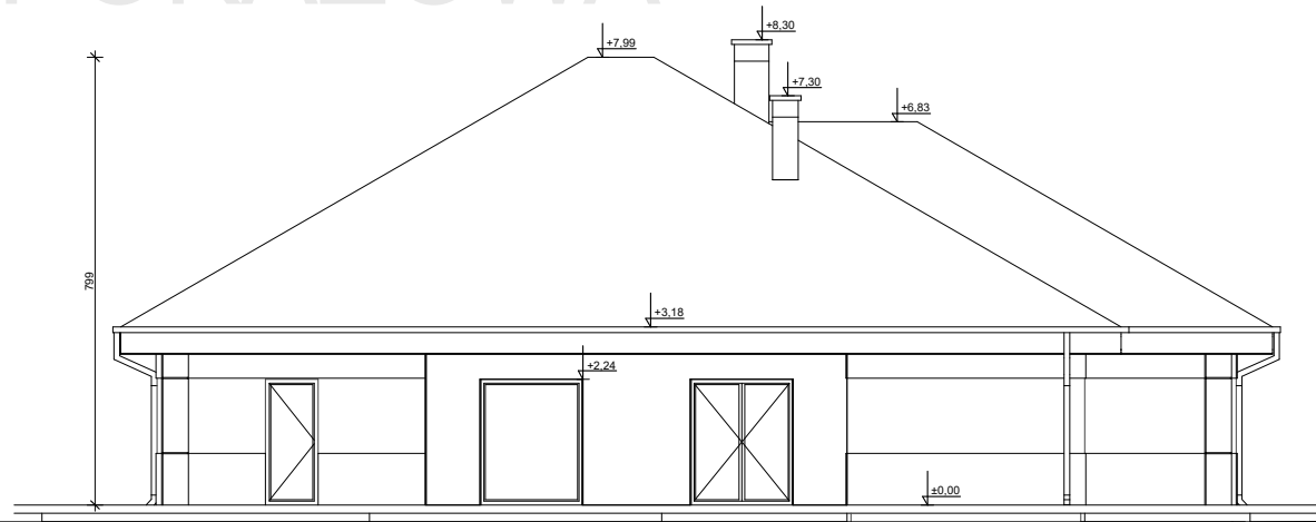
ELEWACJA BOK 1
