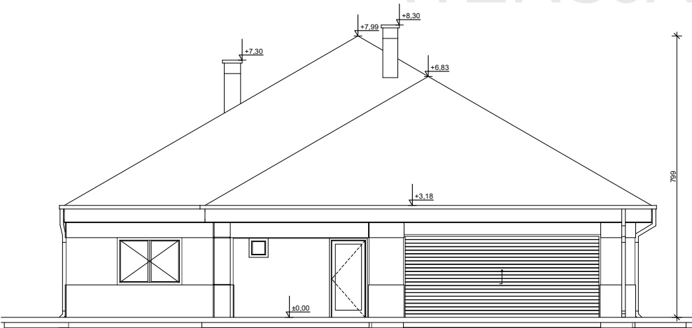
ELEWACJA FRONTOWA
