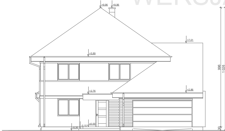
ELEWACJA FRONTOWA
