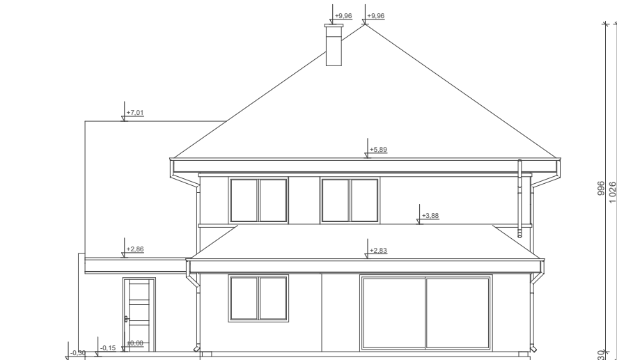
ELEWACJA OGRODOWA
