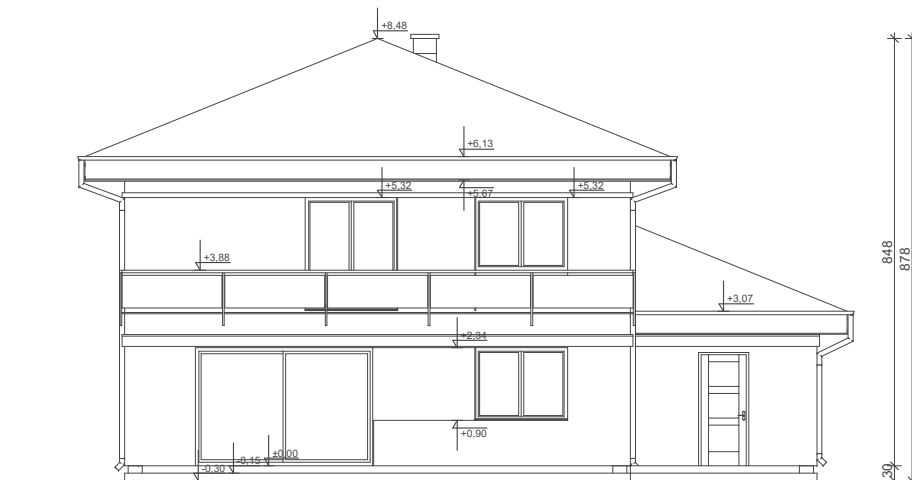
ELEWACJA OGRODOWA
