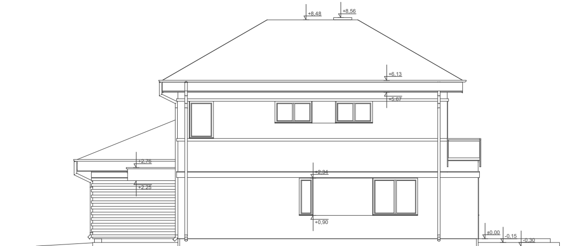
ELEWACJA BOK 2
