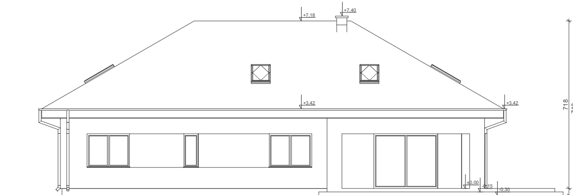
ELEWACJA OGRODOWA
