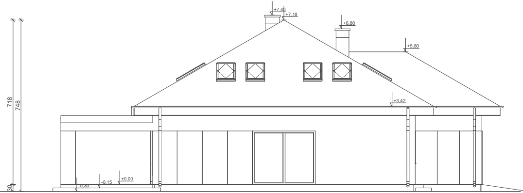
ELEWACJA BOK 1
