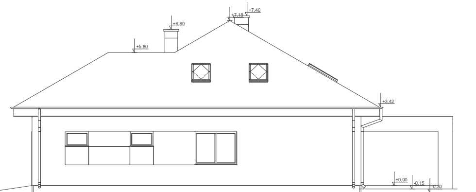
ELEWACJA BOK 2
