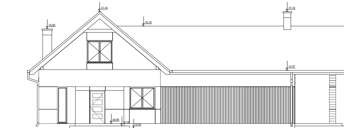
ELEWACJA FRONTOWA
