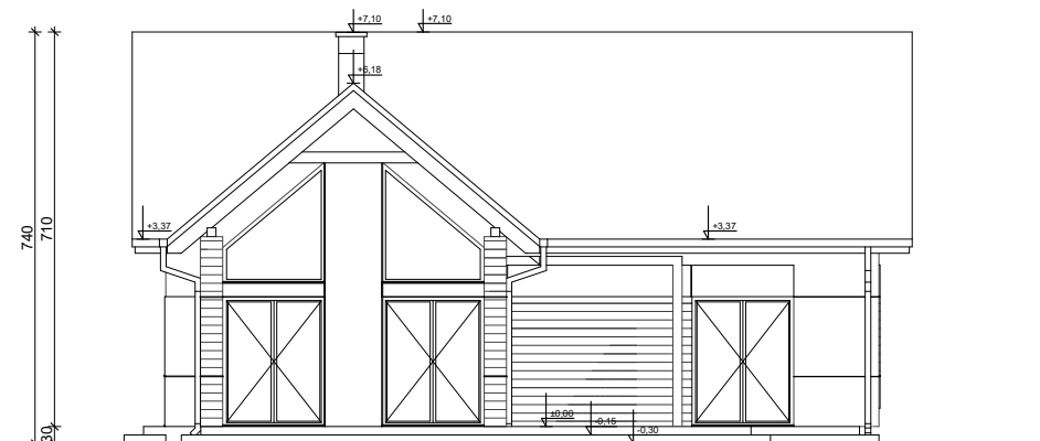
ELEWACJA BOK 2
