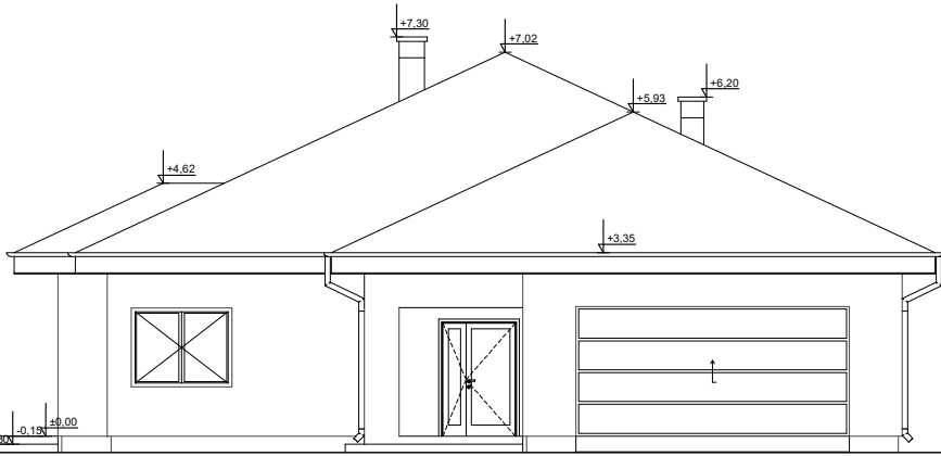
ELEWACJA FRONTOWA
