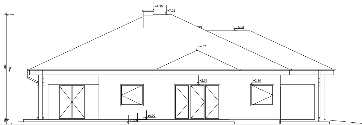
ELEWACJA BOK 1
