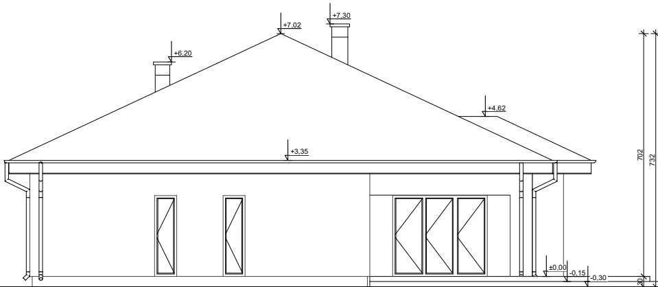
ELEWACJA OGRODOWA
