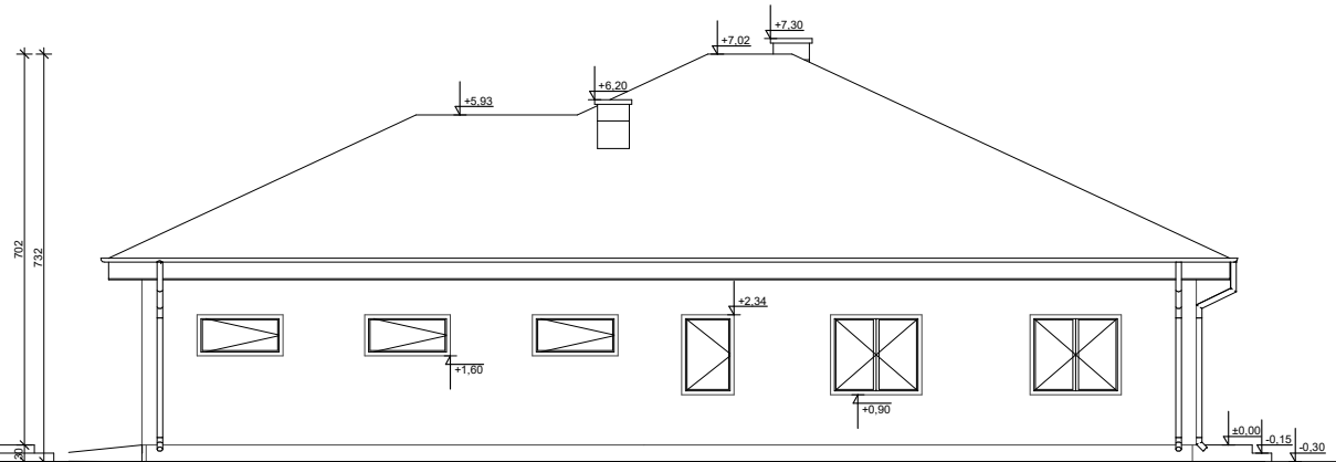
ELEWACJA BOK 2
