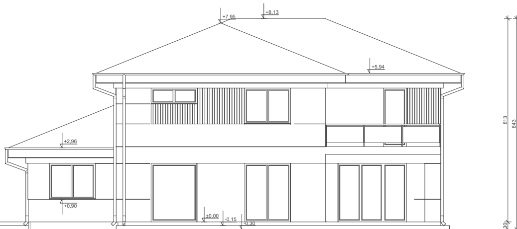
ELEWACJA OGRODOWA
