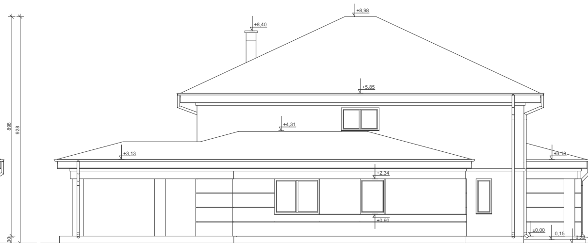
ELEWACJA BOK 2
