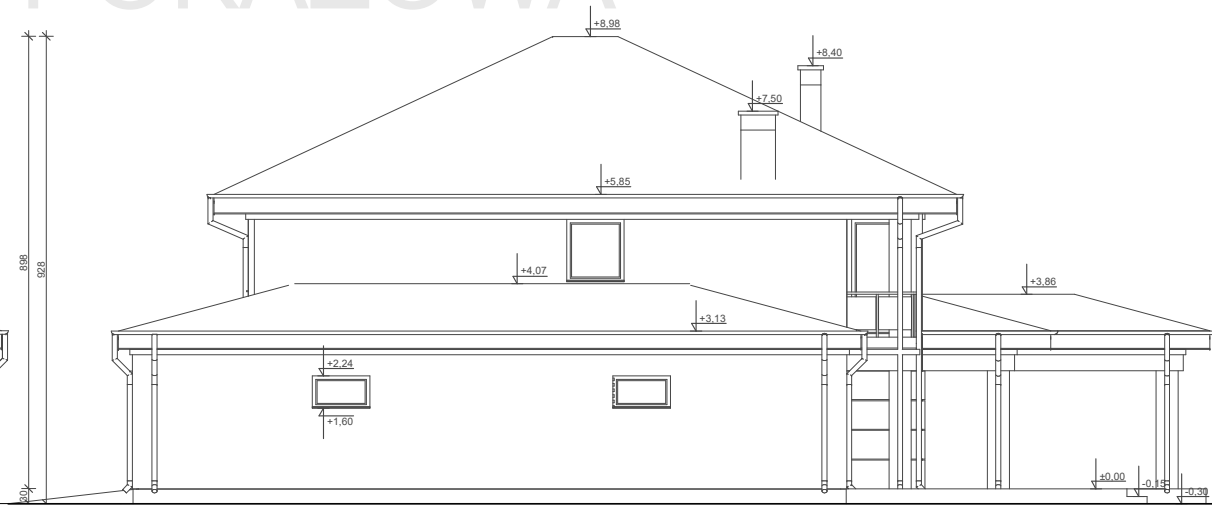
ELEWACJA BOK 1
