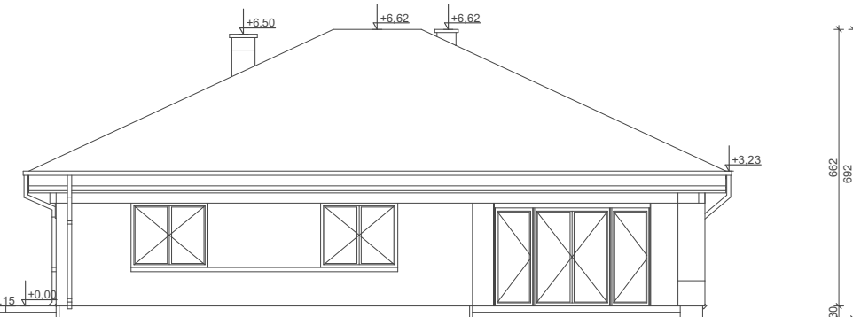
ELEWACJA OGRODOWA
