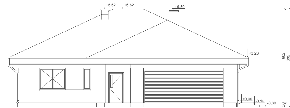
ELEWACJA FRONTOWA
