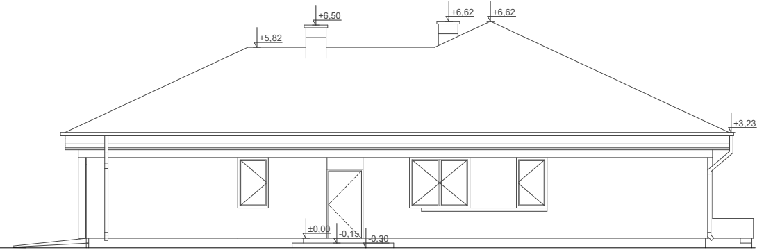
ELEWACJA BOK 1
