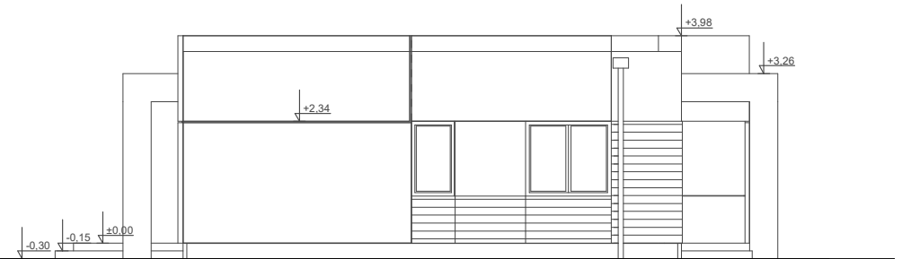
ELEWACJA BOK 1
