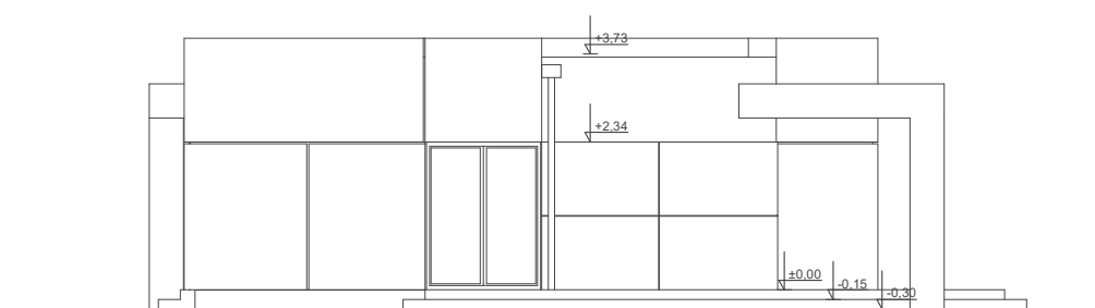
ELEWACJA BOK 2
