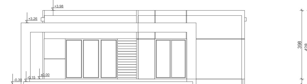
ELEWACJA OGRODOWA
