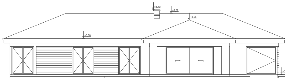
ELEWACJA OGRODOWA
