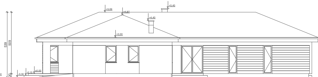
ELEWACJA BOK 2
