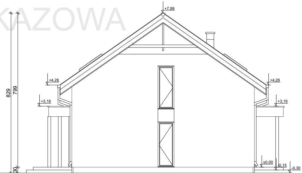
ELEWACJA BOK 1
