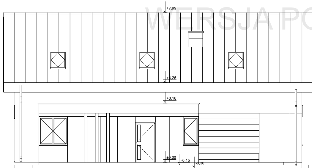
ELEWACJA FRONTOWA
