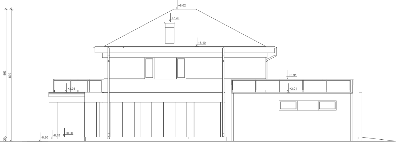
ELEWACJA BOK 1
