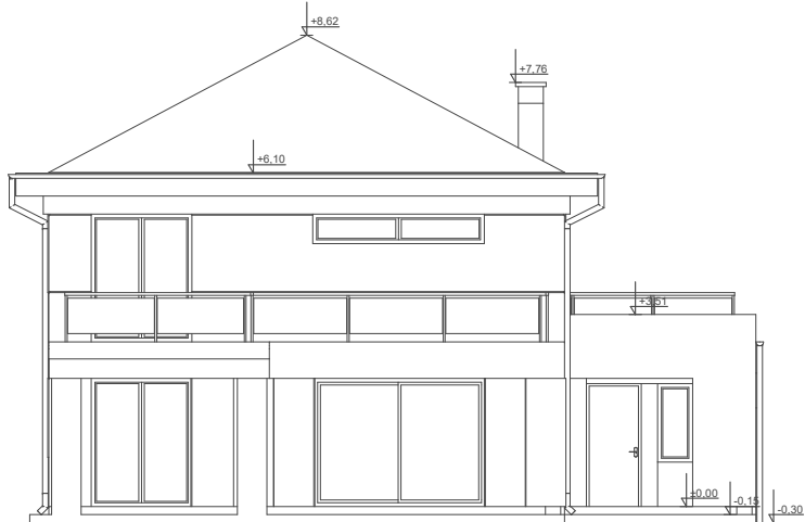
ELEWACJA OGRODOWA
