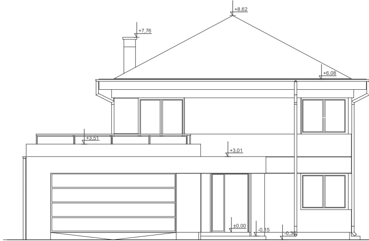
ELEWACJA FRONTOWA
