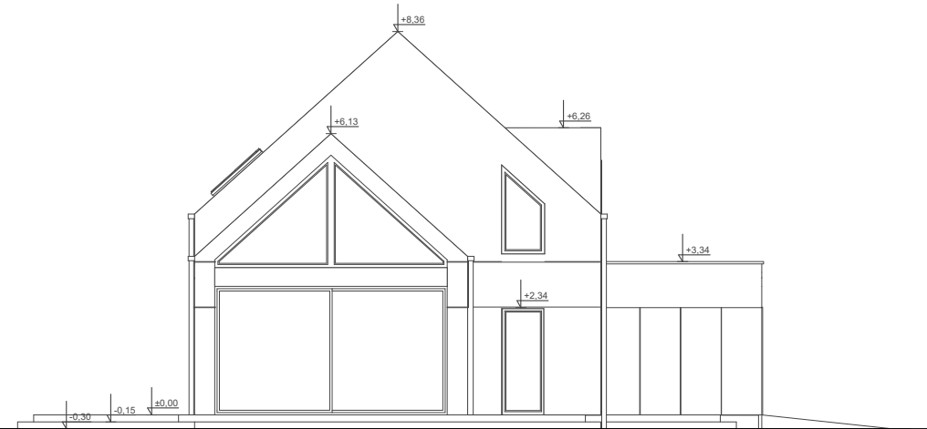
ELEWACJA BOK 1
