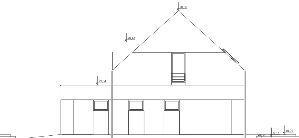
ELEWACJA BOK 2
