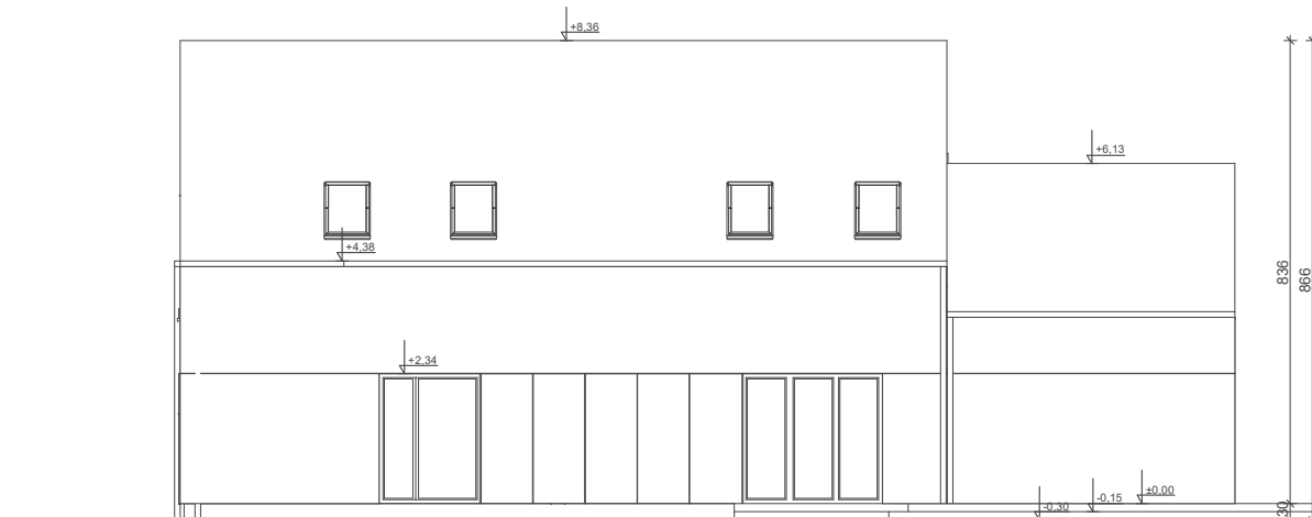
ELEWACJA OGRODOWA
