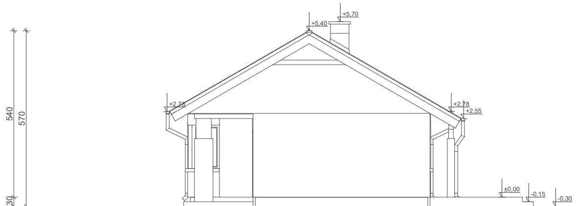
ELEWACJA BOK 2
