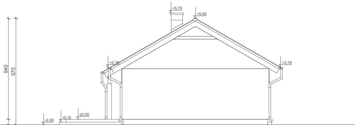
ELEWACJA BOK 1
