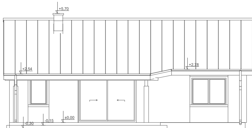
ELEWACJA OGRODOWA
