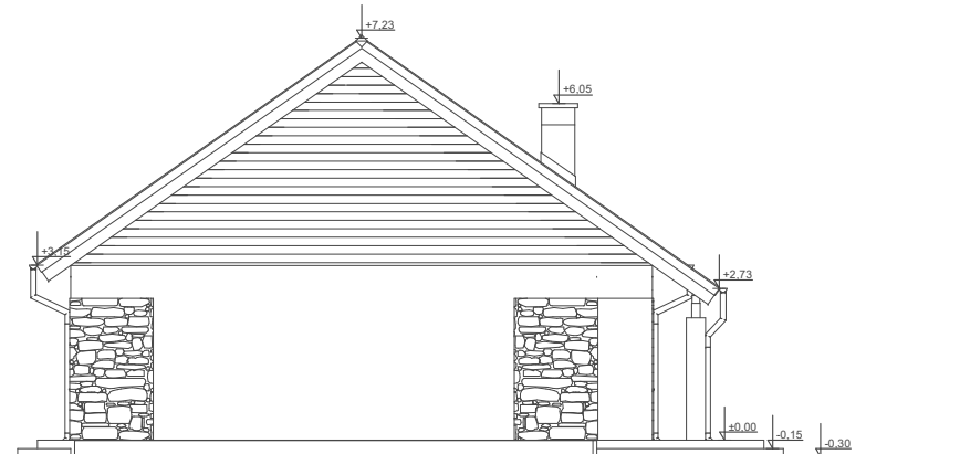
ELEWACJA BOK 2
