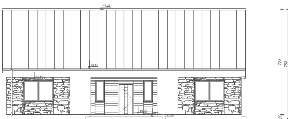
ELEWACJA FRONTOWA
