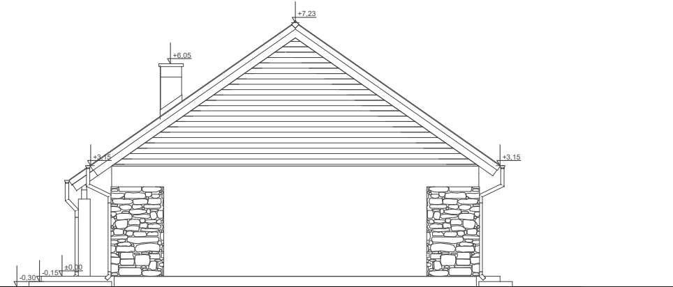
ELEWACJA BOK 1
