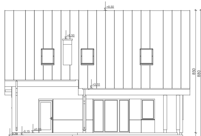
ELEWACJA OGRODOWA
