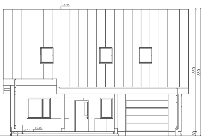
ELEWACJA FRONTOWA
