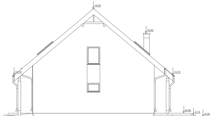
ELEWACJA BOK 2
