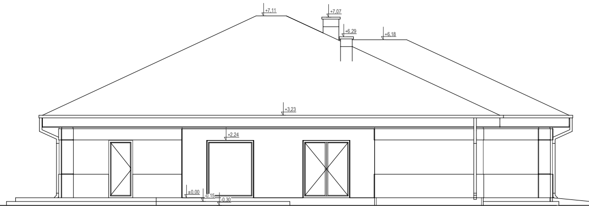
ELEWACJA BOK 1
