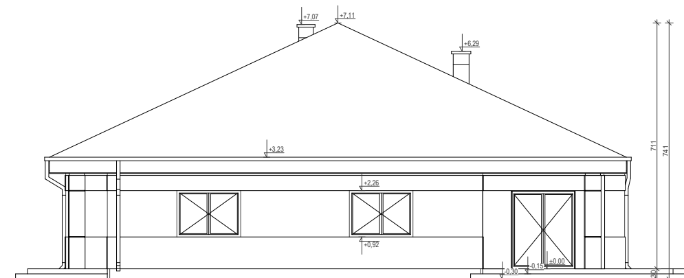
ELEWACJA OGRODOWA
