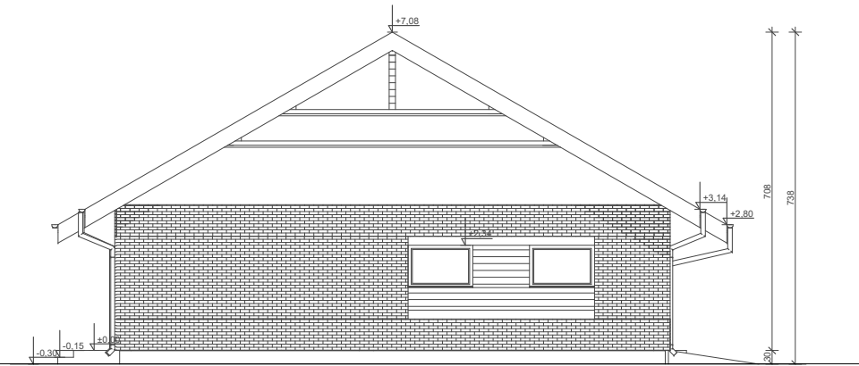
ELEWACJA BOK 1
