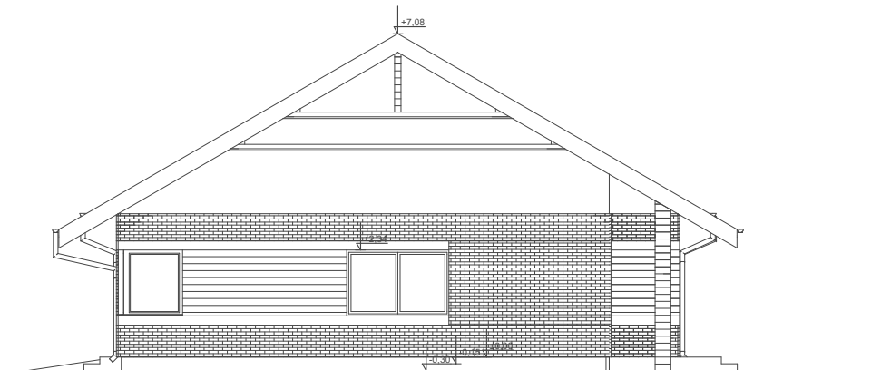
ELEWACJA BOK 2
