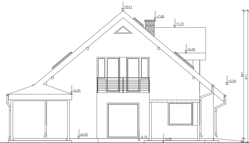
ELEWACJA BOK 1
