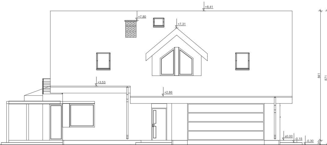
ELEWACJA FRONTOWA
