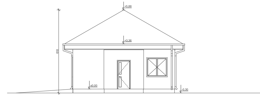
ELEWACJA BOK 2
