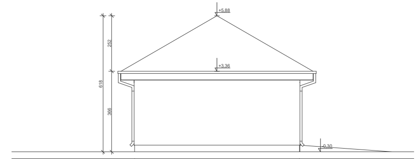
ELEWACJA BOK 1
