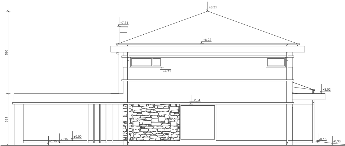
ELEWACJA BOK 1
