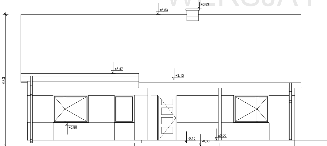
ELEWACJA FRONTOWA
