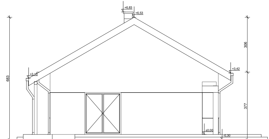
ELEWACJA BOK 2
