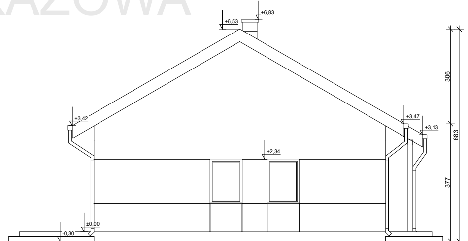
ELEWACJA BOK 1
