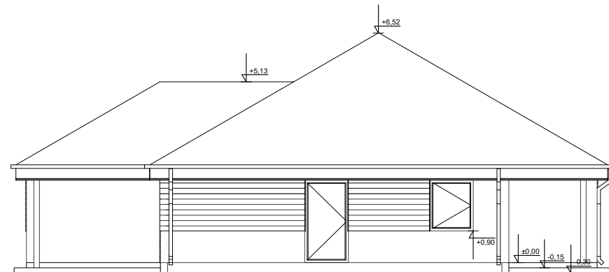
ELEWACJA BOK 2
