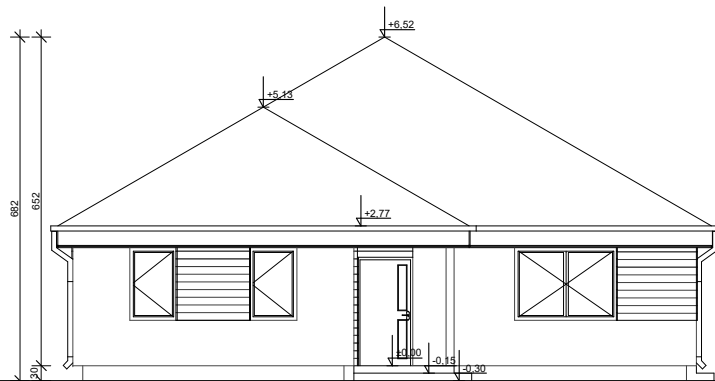
ELEWACJA FRONTOWA
