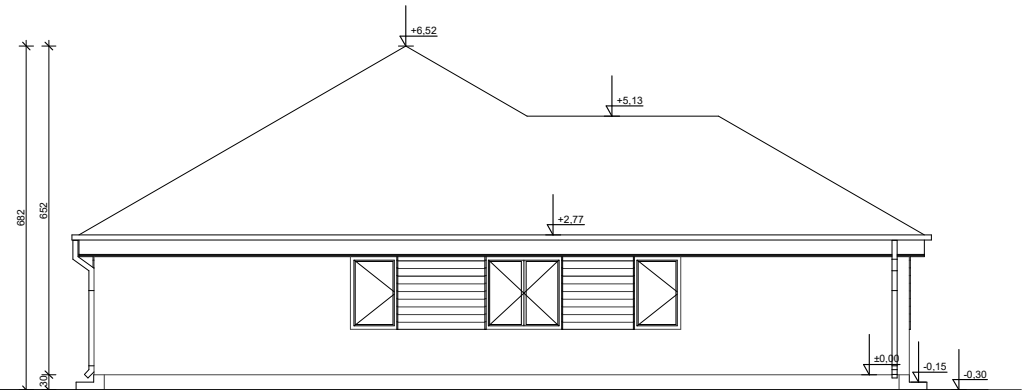
ELEWACJA BOK 1
