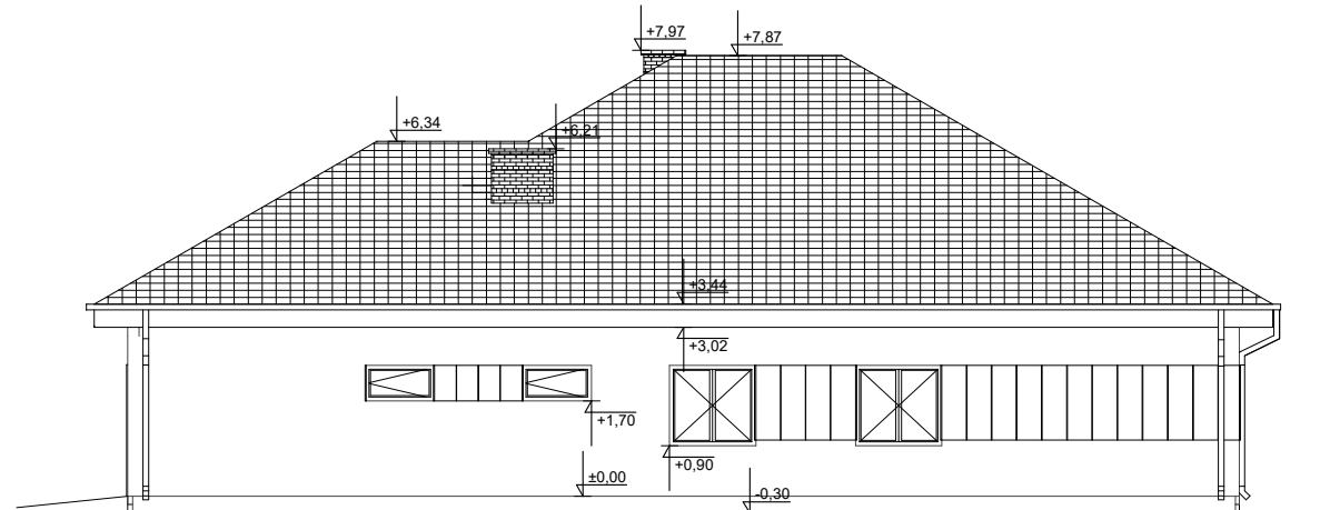
ELEWACJA BOK 2
