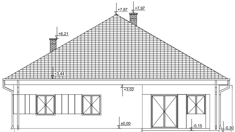
ELEWACJA OGRODOWA
