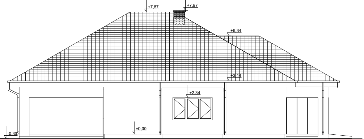
ELEWACJA BOK 1
