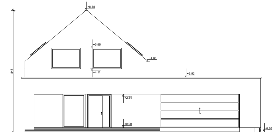
ELEWACJA FRONTOWA
