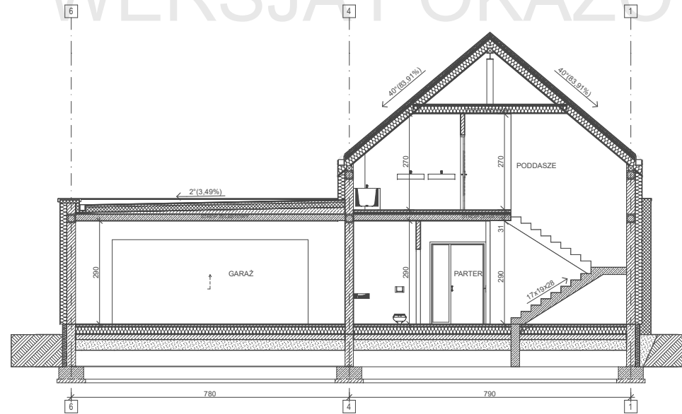
PRZEKROJÓJ A-A
