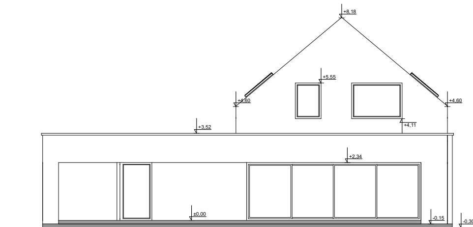
ELEWACJA OGRODOWA
